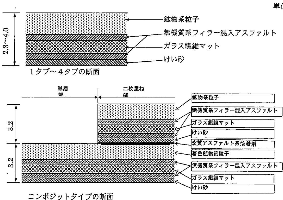
図2 アスファルトシングルの断面構成
