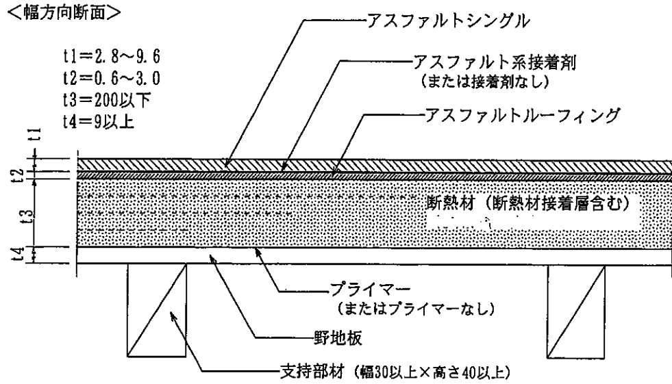
図3 構造説明図
