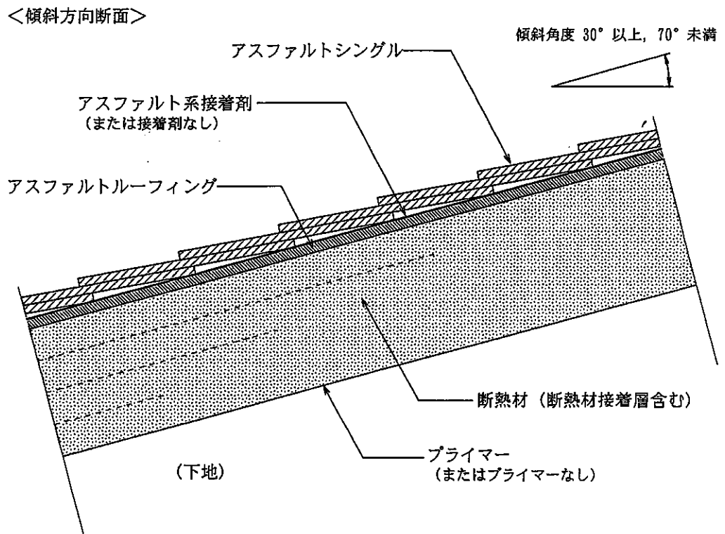
図3 構造説明図
