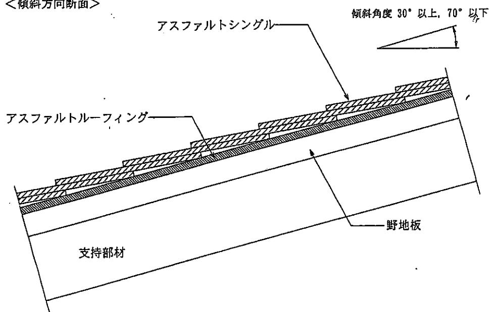
図 4 申請仕様の施工図
