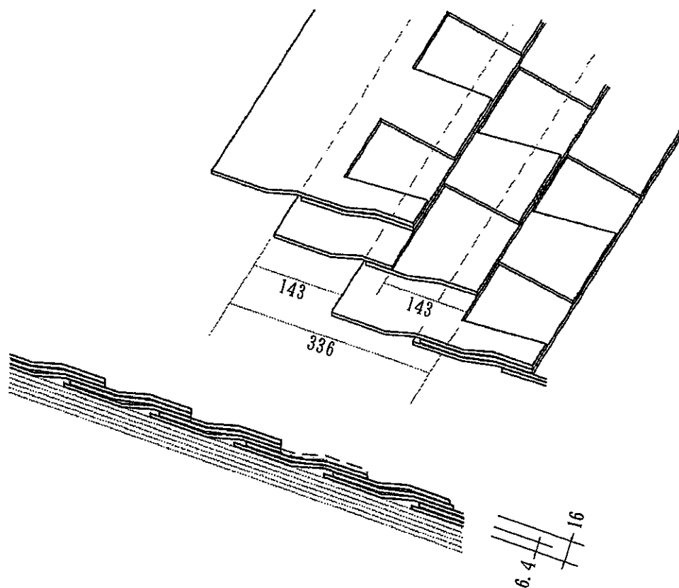
図6 申請仕様の施工図 (アスファルトシングルの施工: コンポジットタイプ)
