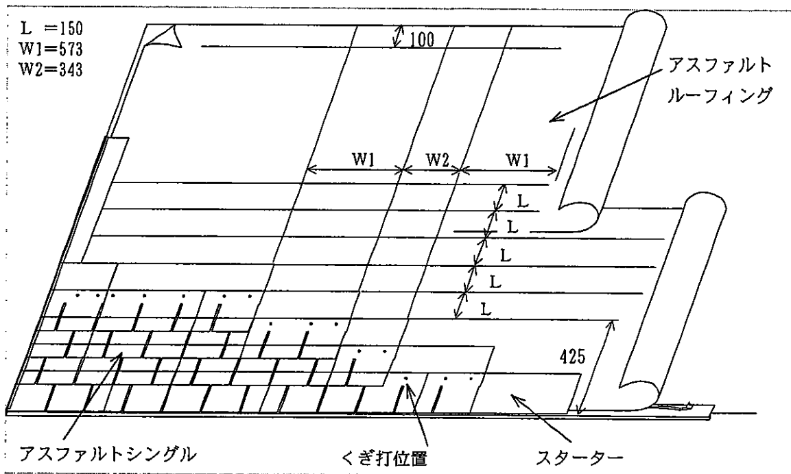
図6 申請仕様の施工図 (アスファルトシングル施工: 1タブ~4タブ)
