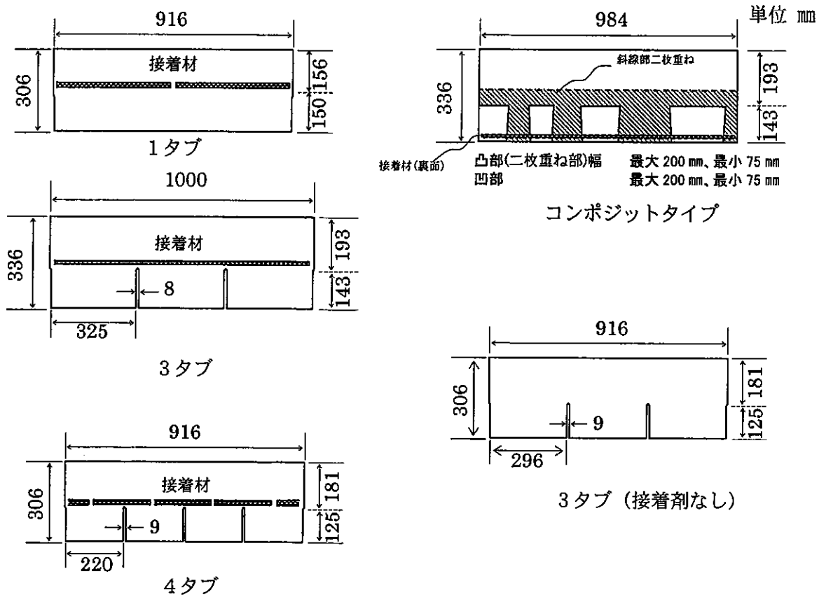
図1 アスファルトシングルの形状
