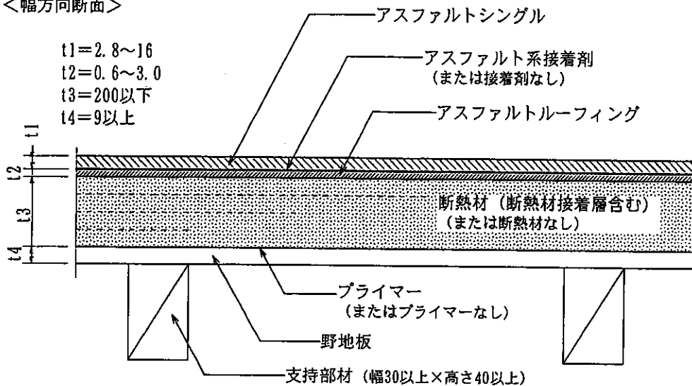
図3 構造説明図
