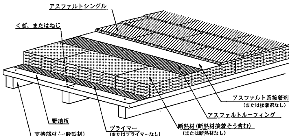
図5 申請仕様の施工図
