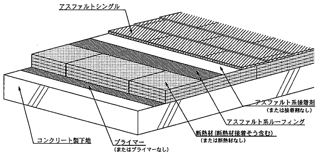
図5 申請仕様の施工図
